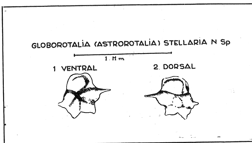
Abb. 1 - Eine neue Art von Globorotalia Cushman
